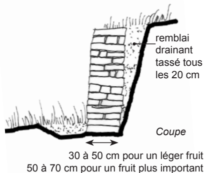
Mur de soutènement en pierre sèche
